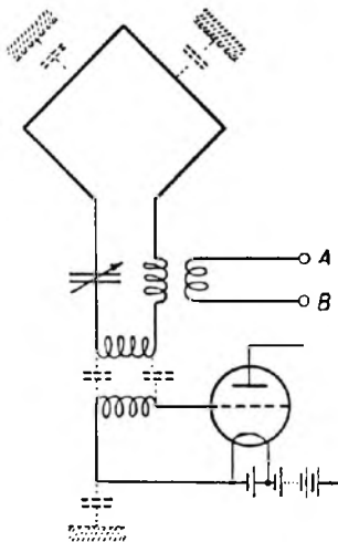
Fig. 2. Normale raamschakeling met compensatie-koppeling
