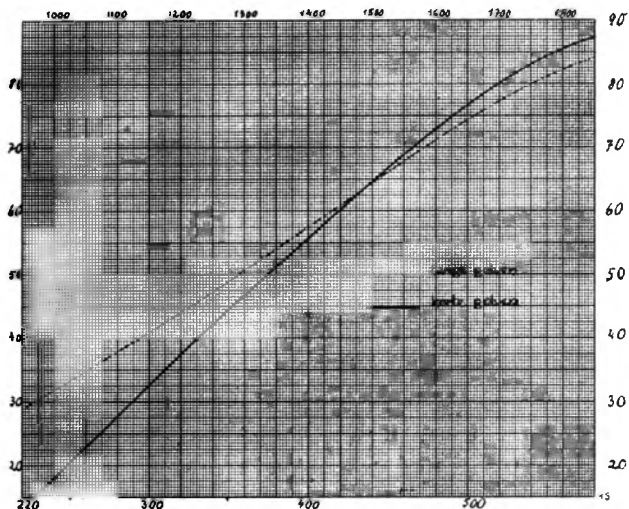
Afstemkrommen van den 1929 Solodyne
